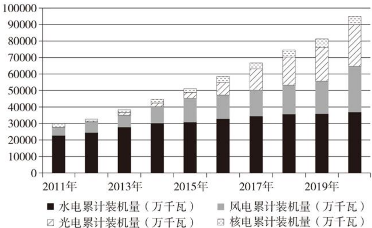
图 2 2011—2020 年中国非化石能源发电装机容量
